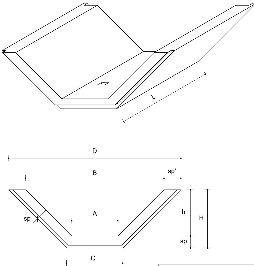
CUNETTA O FOSSA DI GUARDIA A SEZIONE TRAPEZOIDALE
